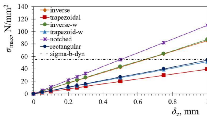
Slika 4.7 Napreznje na savijanje varijacijom različitih vrijednosti progiba vrha konzole na piezoelektričnim konzolnim gredicama [31]
