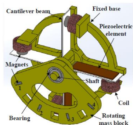
Slika 3.9 Piezoelektromagnetski višesmjerni vibracijski uređaj [33]
