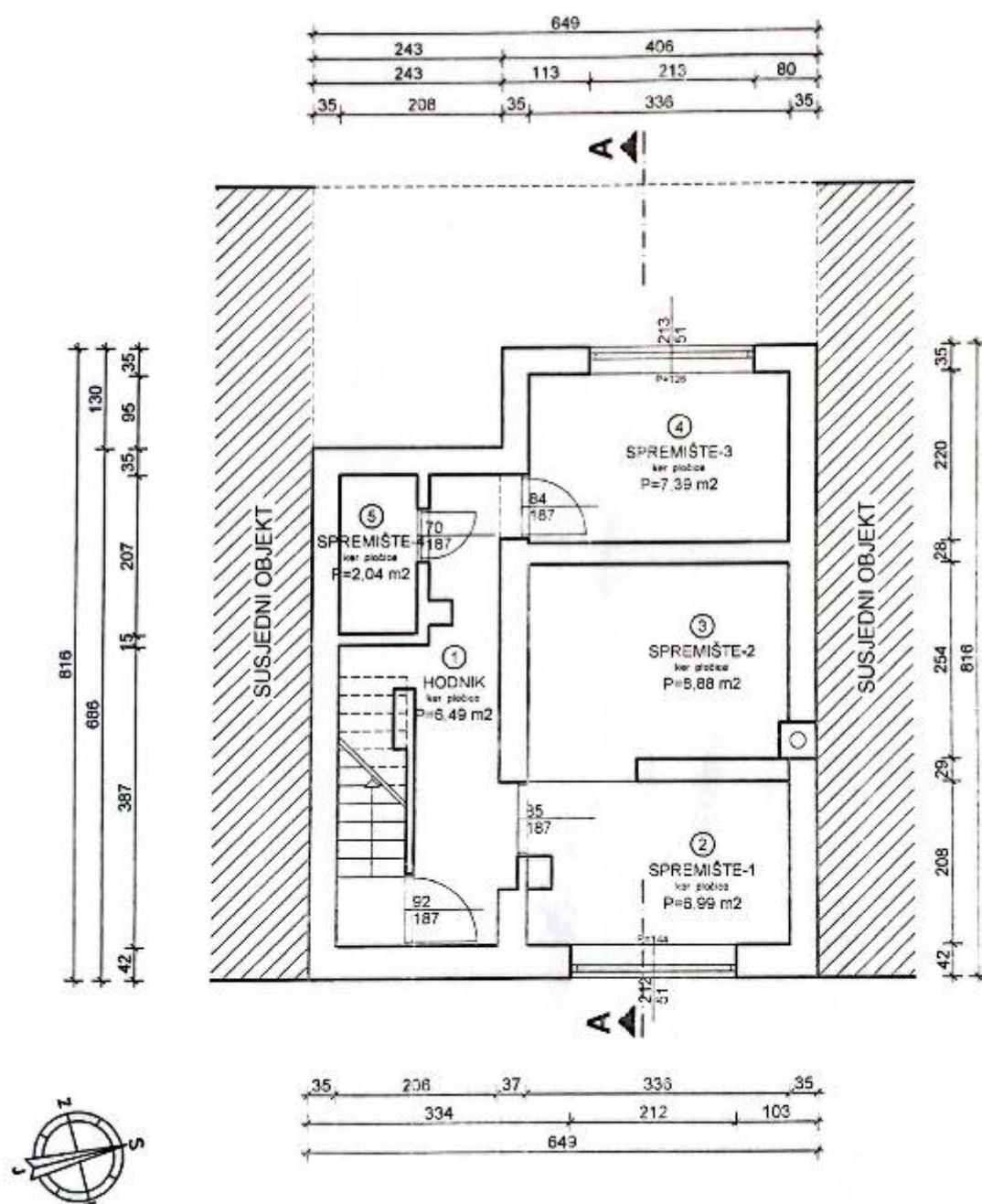
Slika 2.1: Tlocrt podruma
