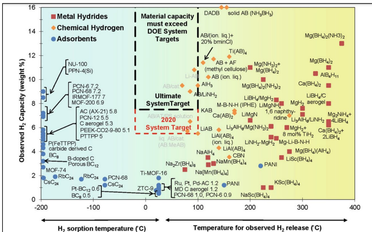
Slika 3.9 Spojevi vodika i veza njihove sorpcije i otpuštanja vodika [1].
