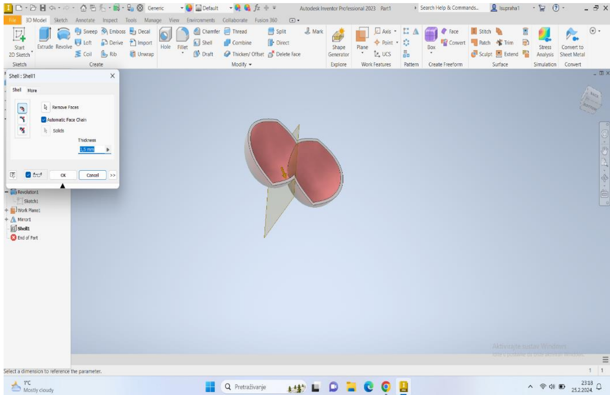
Slika 7.5. Naredba „shell“
