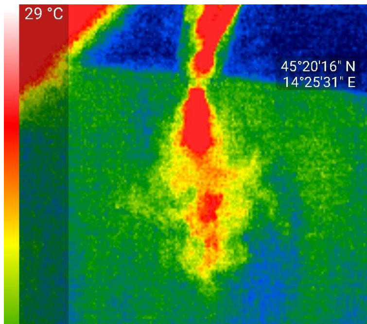
Slika 3.9.: Snimka zabilježena termalnom kamerom prilikom pripreme i provjere opreme
