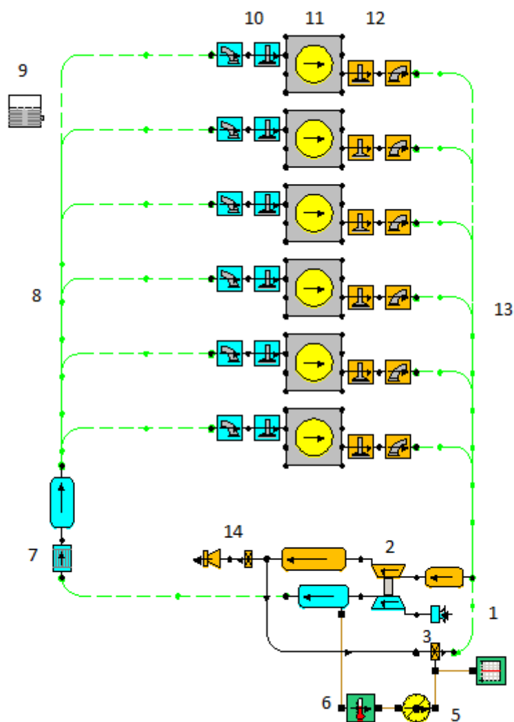
Slika 5.2 Model motora u varijanti prednabijanja s jednim turbopuhalom
