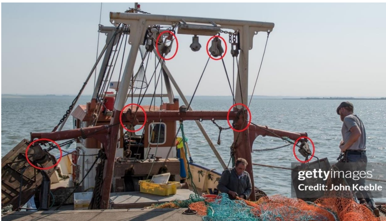
Slika 4.12.3 Primjer koloturnika na kočaru [76]
