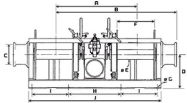
Slika 4.12.2 Osnovne dimenzije odabranog vitla za povlačenje koće [75]
