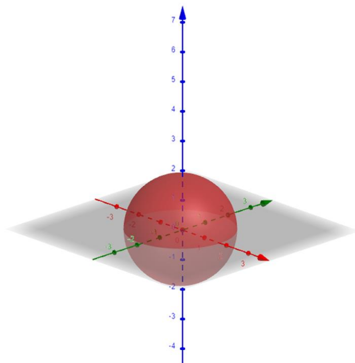
Slika 3.2. Sfera u prostoru [3].
