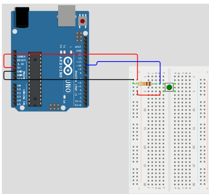
Slika 6.2. Spajanje tipkala u pull-down konfiguraciju.
