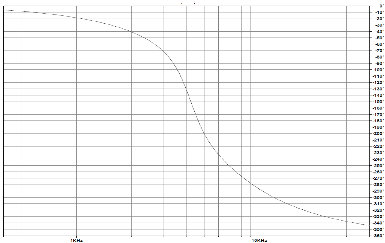
Slika 7.10. Fazno - frekvencijska karakteristika filtra \phi(\omega) .
