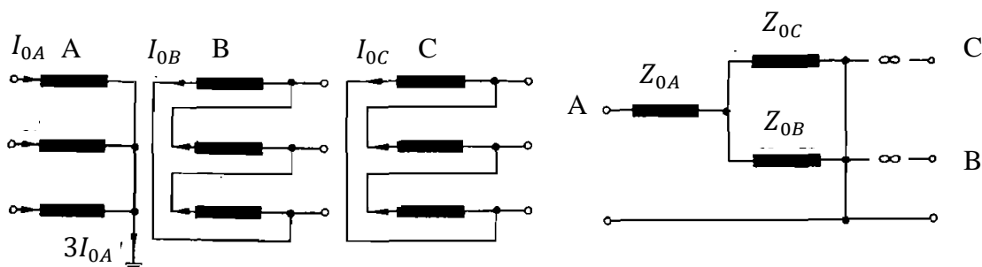
Slika 4.19. Nadomjesna shema spoja zvijezda-trokut-trokut s uzemljenim zvjezdištem [4]
