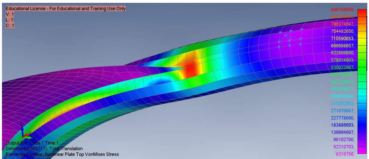
Slika 6.11 Koncentracija naprežanja na modelu s pločastim elementima, test 1
