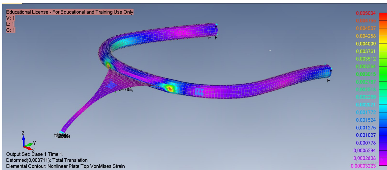
Slika 6.9 Ukupne deformacije modela s pločastim elementima, test 1
