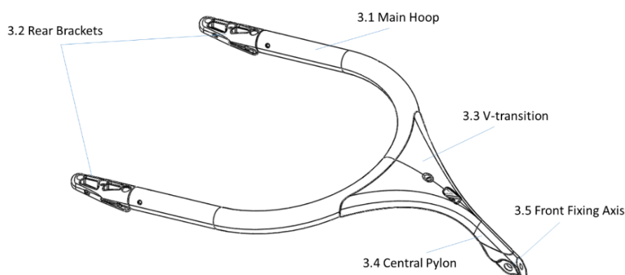
Slika 3.2 Prikaz dijelova koji zajedno čine zavaernu konstrukciju AFP-Halo [11]
