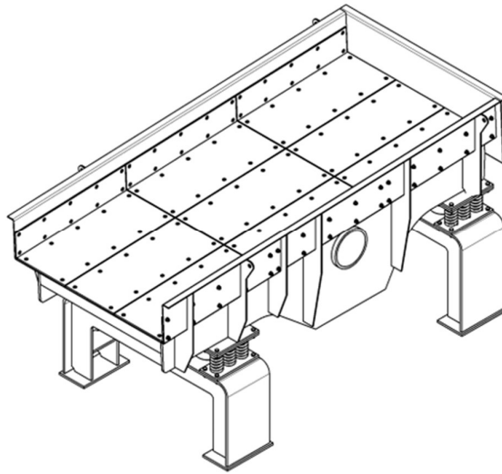
Slika 2.1 Vibrirajući dodavač [1]
