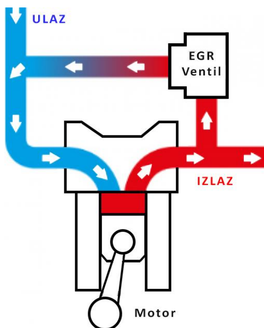
Slika 4.3 Shematski prikaz funkcioniranja EGR sustava
