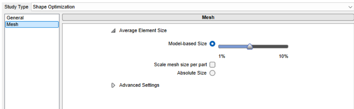
Slika 6.10 Postavke mreže
