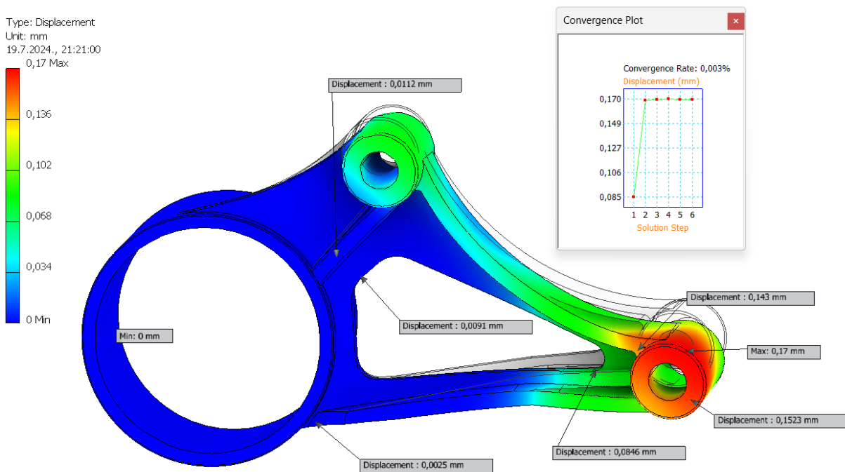
Slika 7.19 Pomaci, model 1
