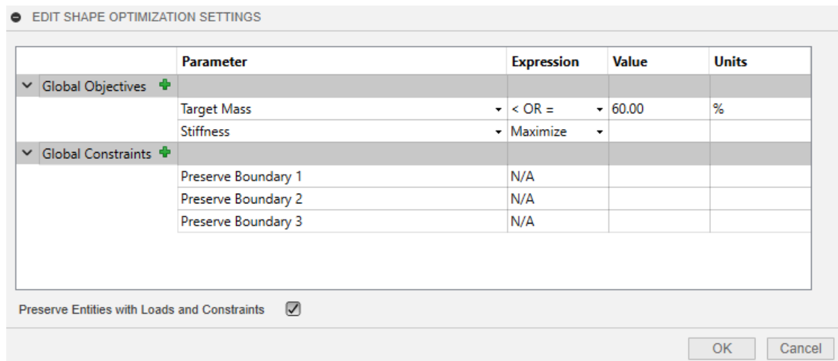
Slika 6.8 Ciljevi optimizacije
