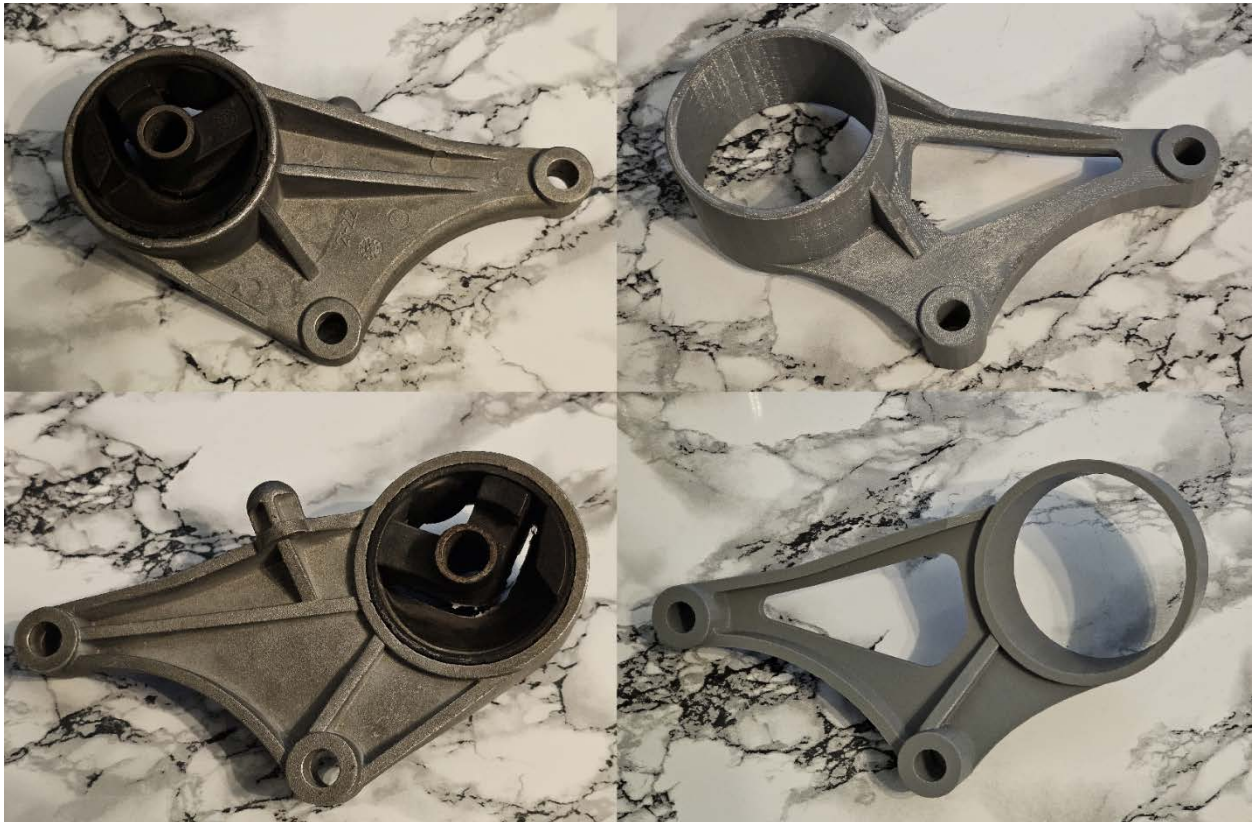
Slika 8.6 Usporedba stvarnog i optimiranog nosača
