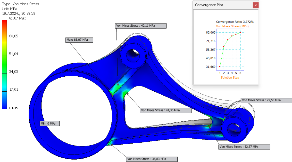
Slika 7.18 Naprezanja prema von Misesu, model 1
