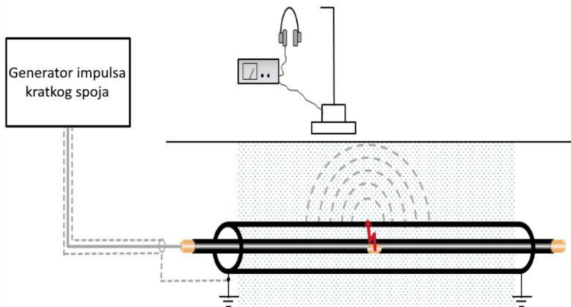
Slika 6.1 Prikaz korištenja akustične metode lokalizacije kvara [2]
