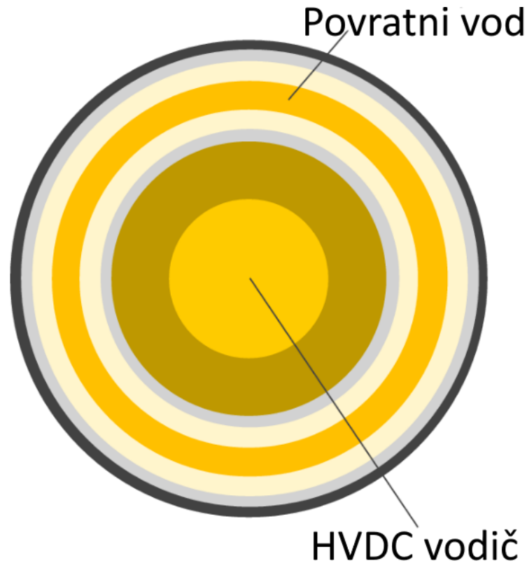
Slika 3.2 Pojednostavljeni prikaz jednožilnog HVDC kabla sa integriranim povratnim vodom [19]
