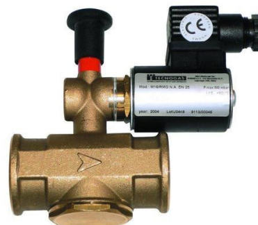
Slika 6.14: Elektromagnetski ventil
