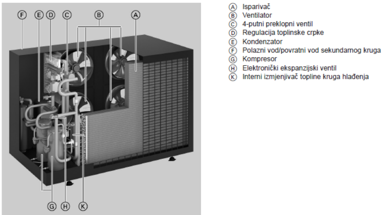
Slika 6.1. Presjek dizalice topline zrak-voda [14]
