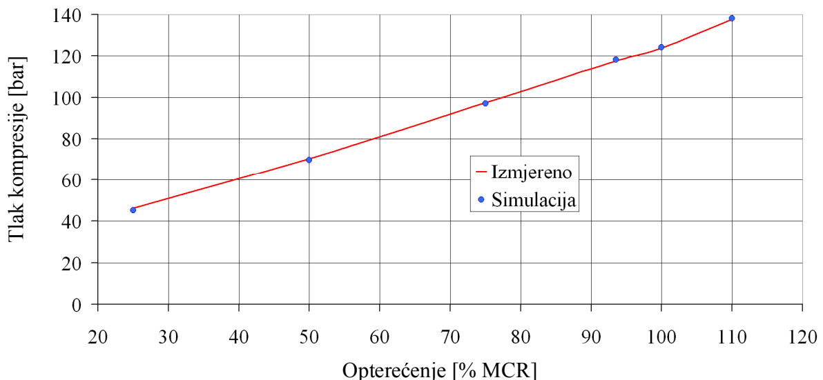
Slika 9.1. Usporedba izmjerena i simulirana tlaka kompresije na motoru MAN 6S50MC
