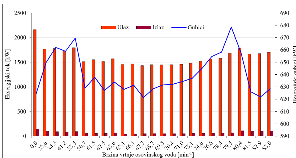
Slika 4.18 Eksergijski tokovi i eksergijski gubici turbogeneratora pri promjeni opterećenja osovinskog voda
