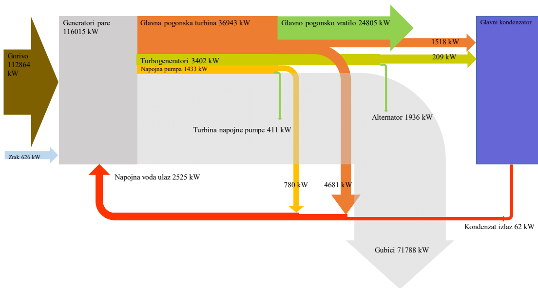
Slika 7.5 Sankeyev diagram parnoturbinskog postrojenja na 83,00 \text{ min}^{-1} , eksergijski tokovi
