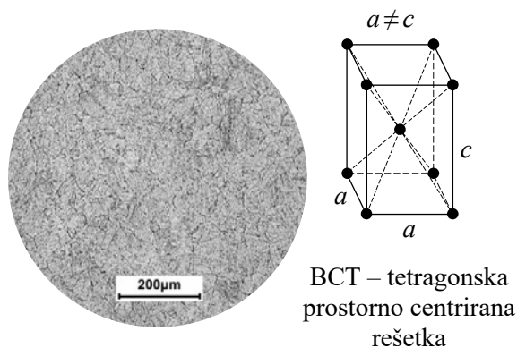
Slika 4.13. Mikrostruktura martenzitnog nehrđajućeg čelika (mikrografija: [11])
