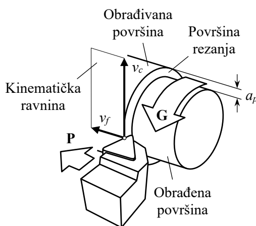
Slika 4.1. Gibanja alata i obratka kod tokarenja. G glavno i P posmično gibanje, a_p dubina rezanja, v_c brzina rezanja, v_f posmična brzina
