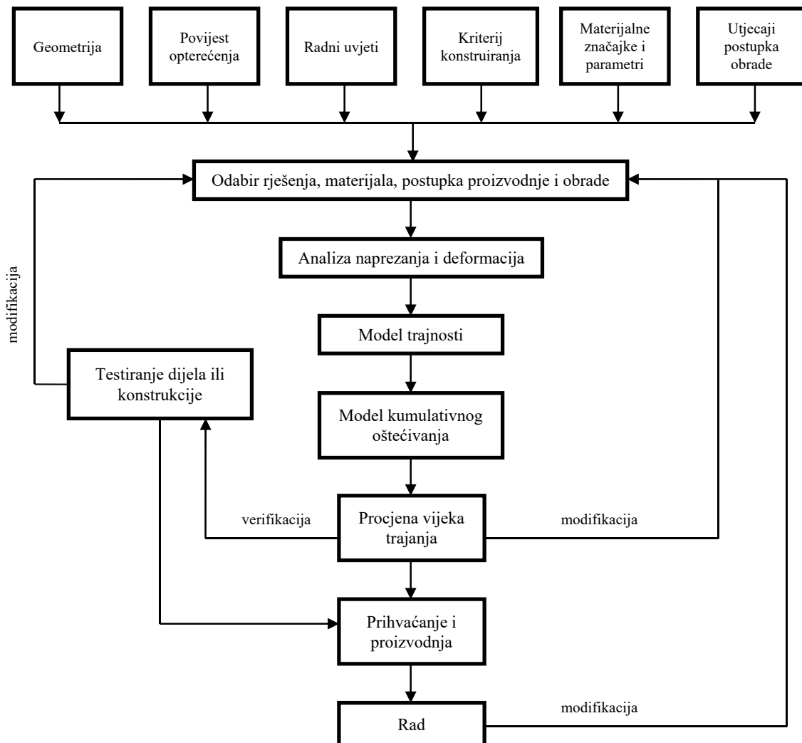
Slika 1.1 Dijagram toka konstruiranja s obzirom na vijek trajanja, prema [78]
