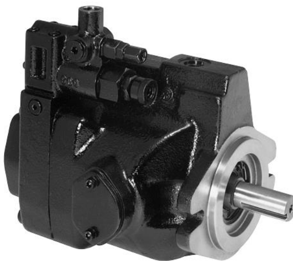
Slika 3-4 Hidraulička pumpa "Parker PVP16"
