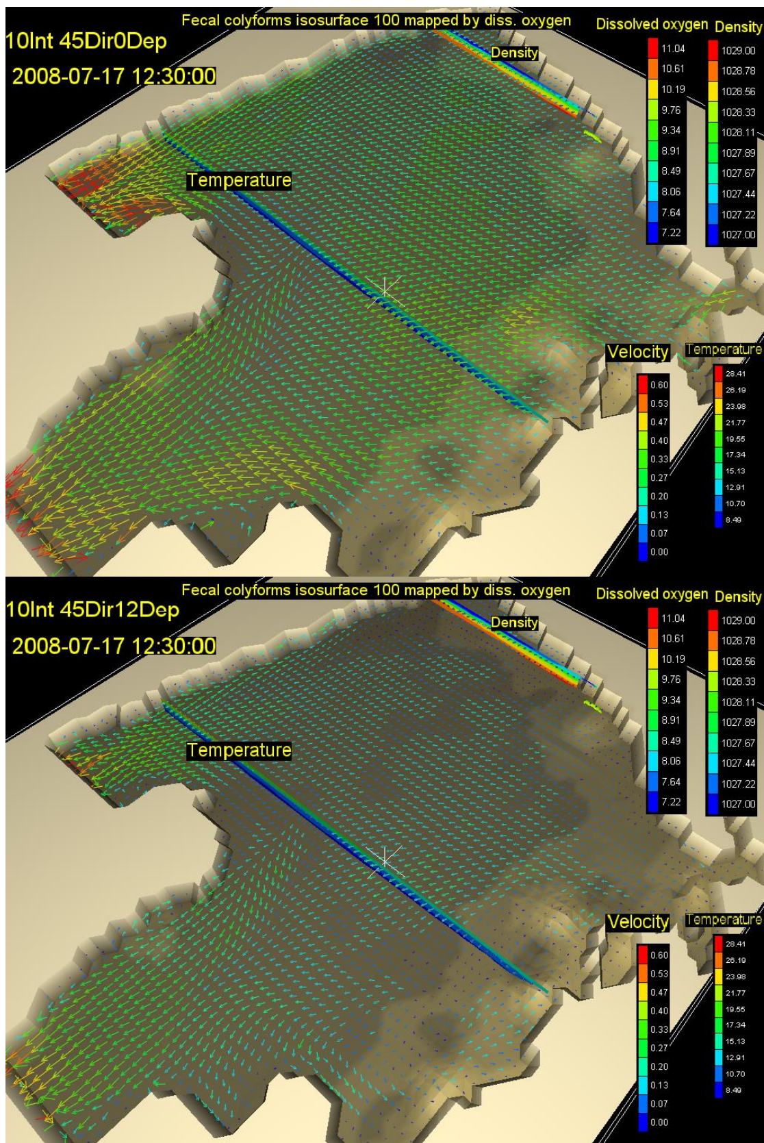
Slika 23. Vektori brzina na površini (gore) i na dubini od 12m (dolje) s vertikalnim profilom gustoće i temperature, te oblakom onečišćenja koncentracije 100 FC(100 ml) -1 za 16,5. st za vjetar intenziteta 10 ms -1 iz smjera 45 stupnjeva
