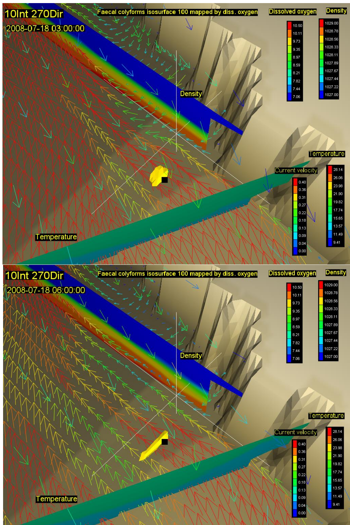
Slika 81. Vektori brzina na površini (rijetki raster) i na dubini od 20m (gusti raster) s vertikalnim profilom gustoće i temperature, te oblakom onečišćenja koncentracije 100 \text{FC}(100 \text{ ml})^{-1} za 33. (gore) i 36. st (dolje) za vjeter intenziteta 10 \text{ ms}^{-1} iz smjera 270 stupnjeva
