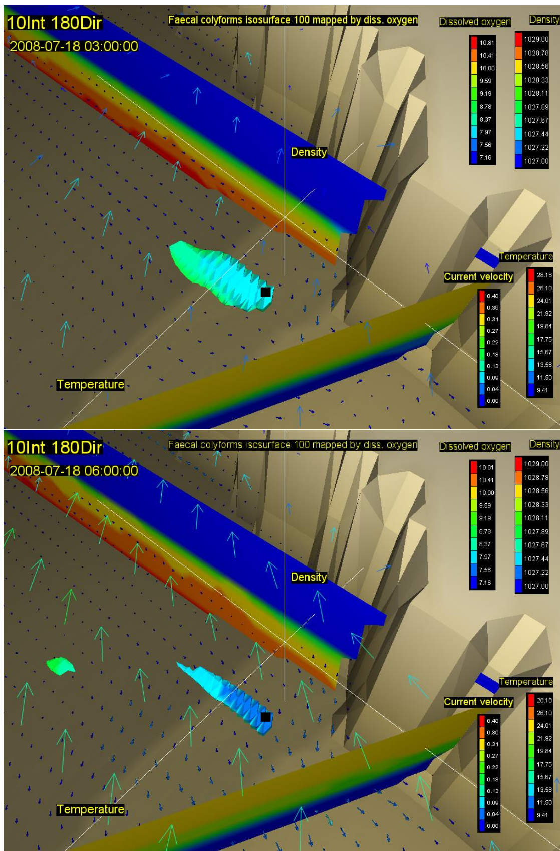
Slika 64. Vektori brzina na površini (rijetki raster) i na dubini od 20m (gusti raster) s vertikalnim profilom gustoće i temperature, te oblak onečišćenja koncentracije 100 FC(100 ml) -1 za 33. (gore) i 36. st (dolje) za vjeter intenziteta 10 ms -1 iz smjera 180 stupnjeva
