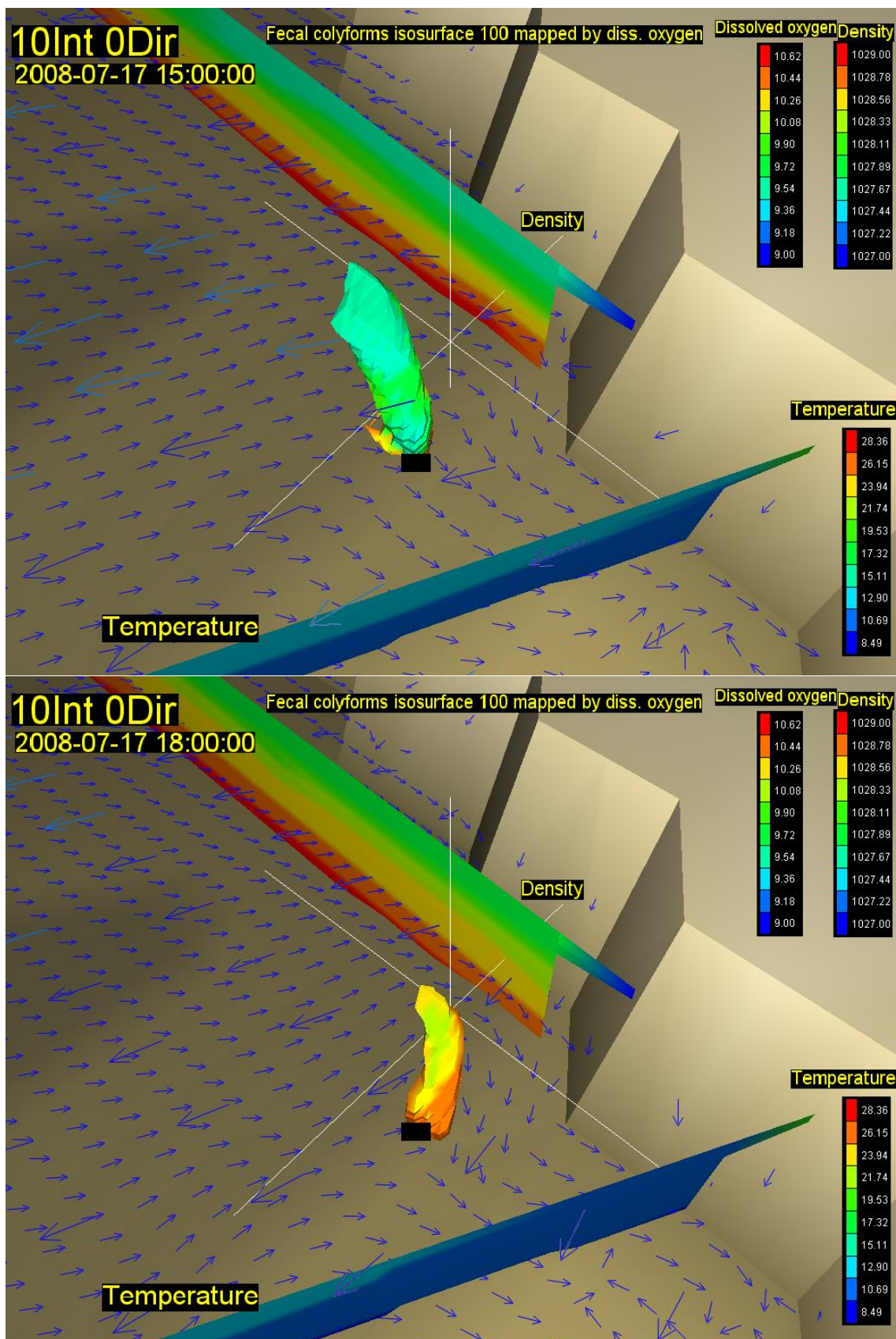
Slika 44. Vektori brzina na površini (rijetki raster) i na dubini od 20m (gusti raster) s vertikalnim profilom gustoće i temperature, te oblakom onečišćenja koncentracije 100 \text{ FC}(100 \text{ ml})^{-1} za 21. (gore) i 24. st (dolje) za vjetar intenziteta 10 \text{ ms}^{-1} iz smjera 0 stupnjeva
