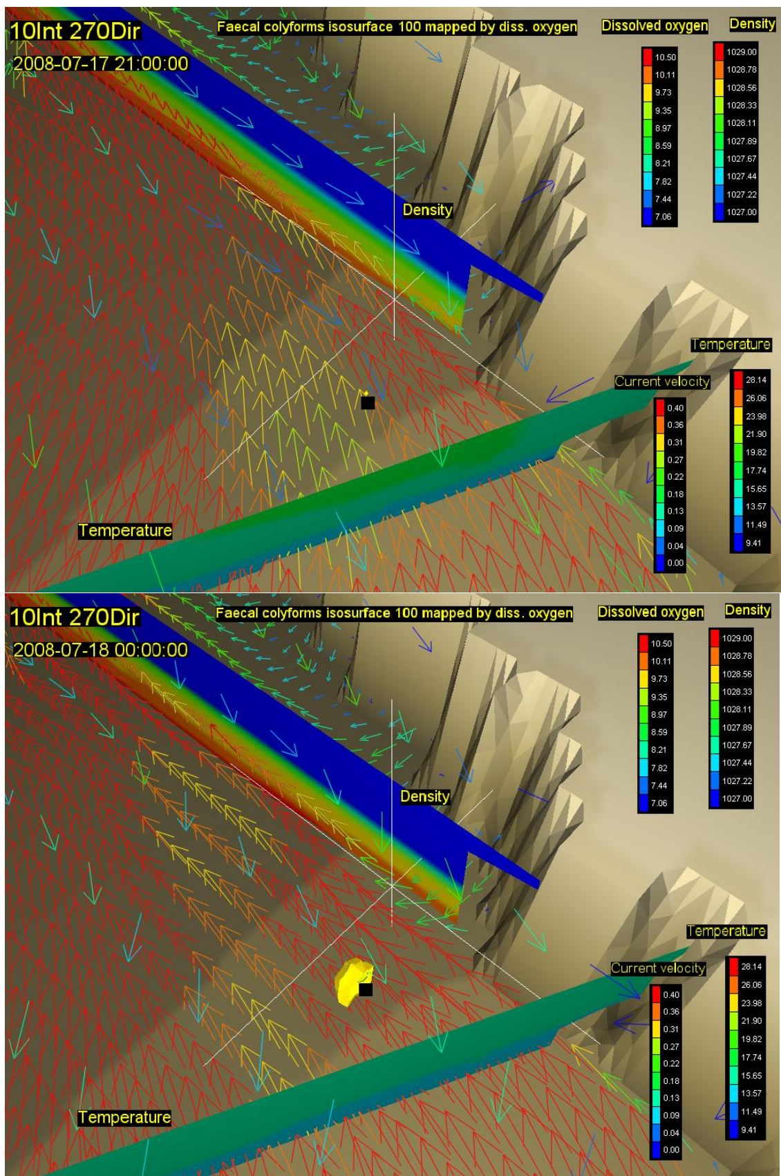
Slika 80. Vektori brzina na površini (rijetki raster) i na dubini od 20m (gusti raster) s vertikalnim profilom gustoće i temperature, te oblakom onečišćenja koncentracije 100 \text{FC}(100 \text{ ml})^{-1} za 27. (gore) i 30. st (dolje) za vjeter intenziteta 10 \text{ ms}^{-1} iz smjera 270 stupnjeva
