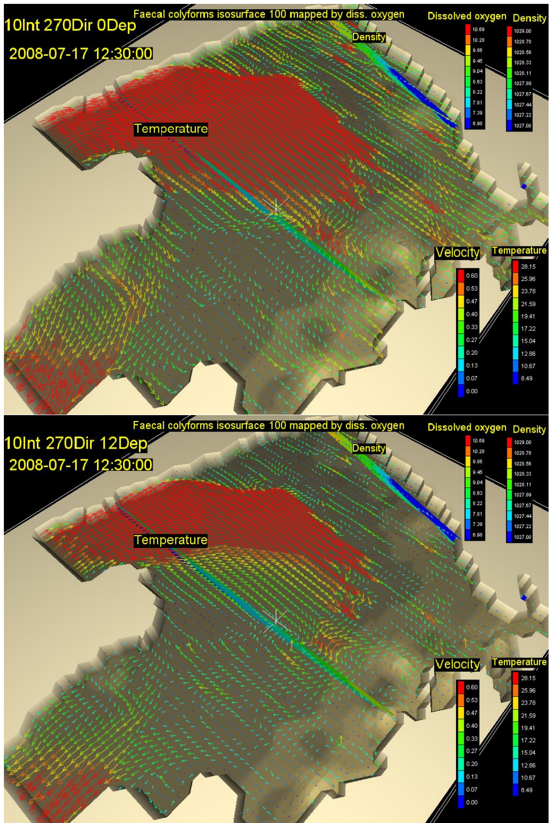
Slika 82. Vektori brzina na površini (gore) i na dubini od 12m (dolje) s vertikalnim profilom gustoće i temperature, te oblakom onečišćenja koncentracije 100 FC(100 ml) -1 za 16,5. st za vjeter intenziteta 10 ms -1 iz smjera 270 stupnjeva
