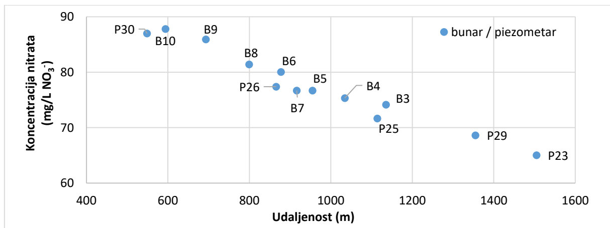
Slika 5-62 Dijagram disperzije: udaljenost - koncentracija nitrata
