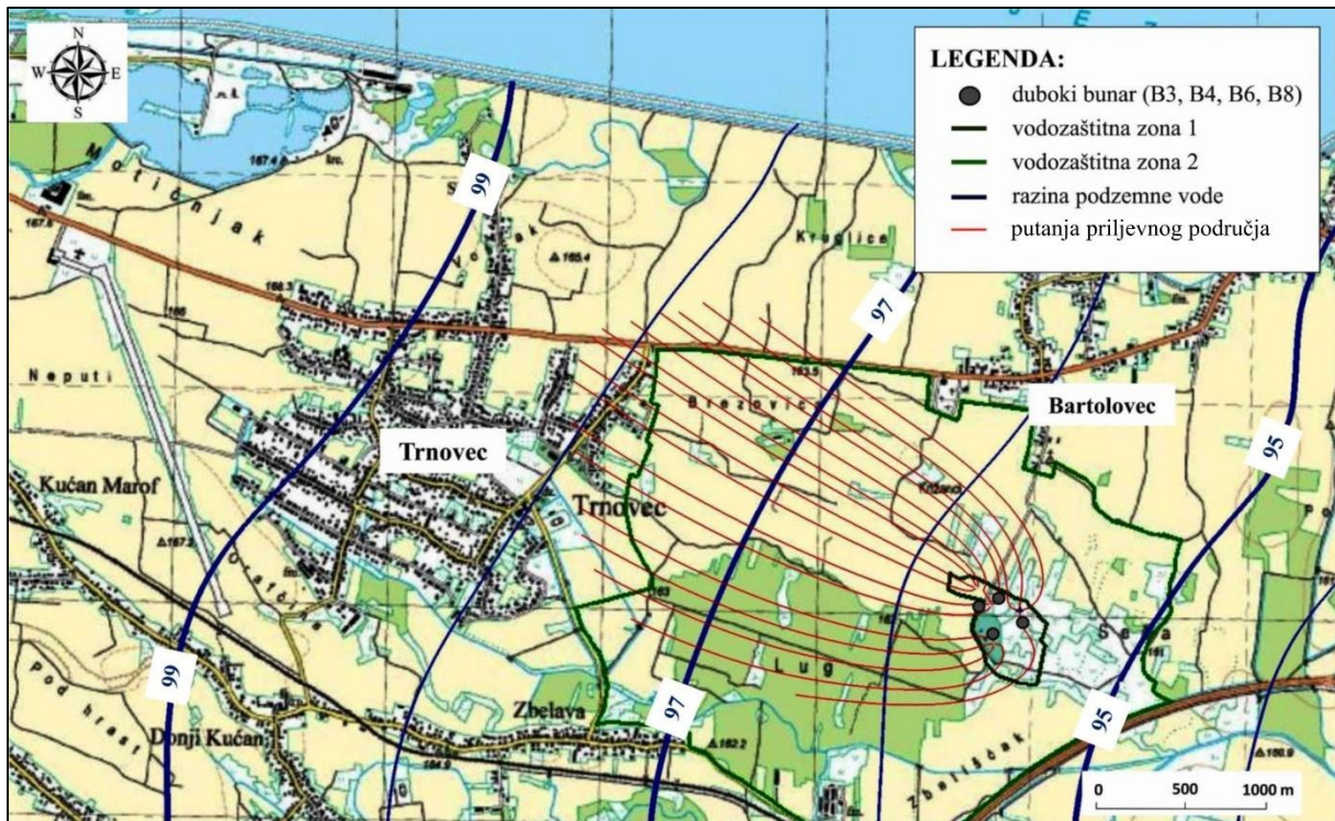
Slika 6-4 Simulacija toka podzemne vode na vodocpilištu Bartolovec 2
