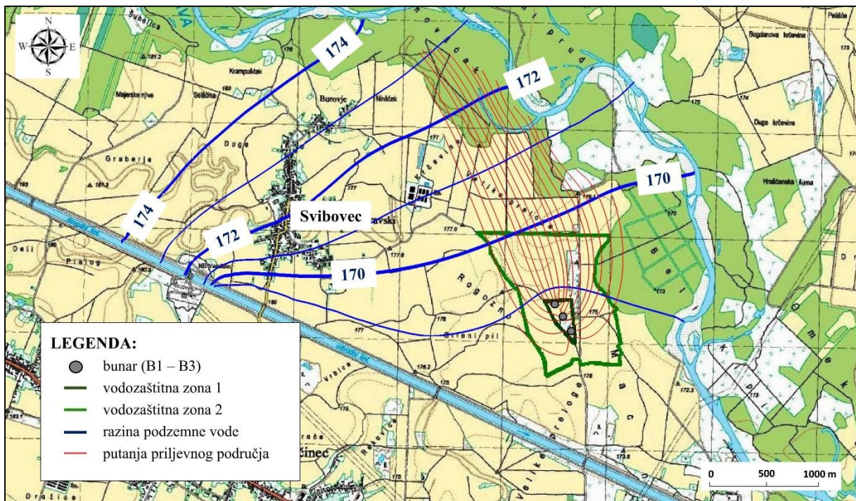
Slika 6-5 Simulacija toka podzemne vode na vodocpilištu Vinokovščak
