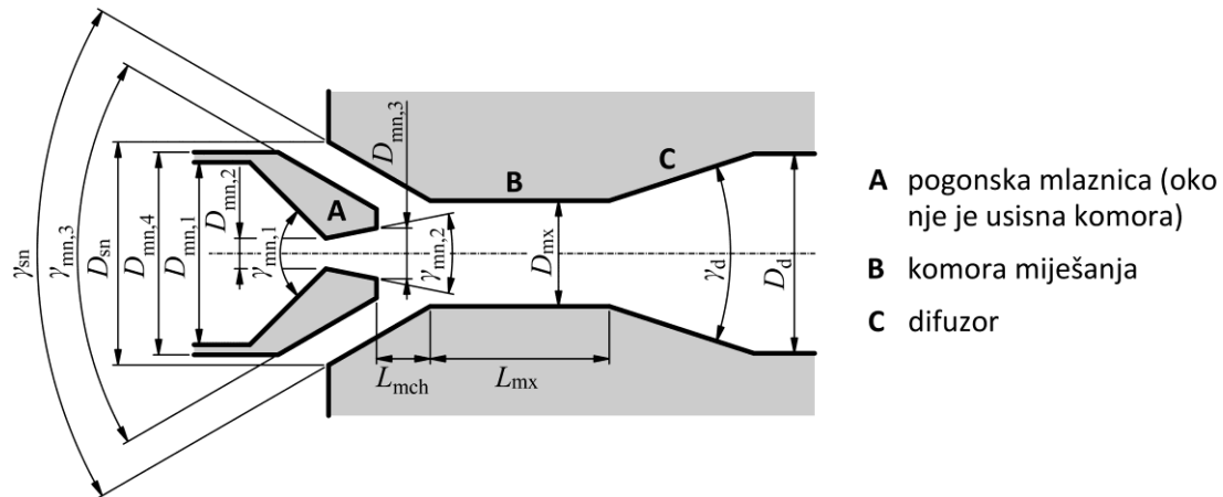
Slika 3.29 Geometrija ejektora
