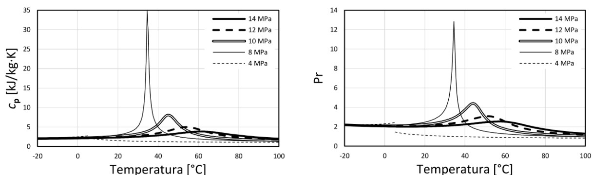
Slika 2.3 Izobarna specifična toplina CO 2 (lijevo) i Prandtlov broj (desno)
