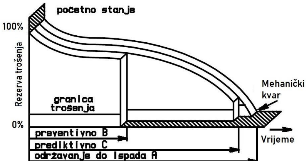
Slika 7.1. Strategije održavanja [1]
