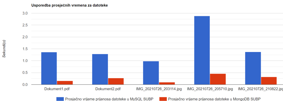
Slika 4.5: Prijenos podataka - prosječno vrijeme prijensa za iste datoteke
