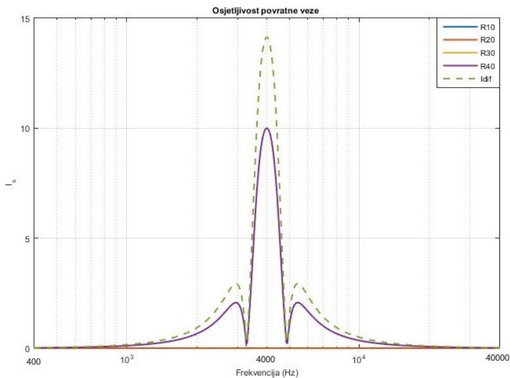
Slika 5.6. Prikaz Schofflerove osjetljivosti povratne veze bikvartne strukture.
