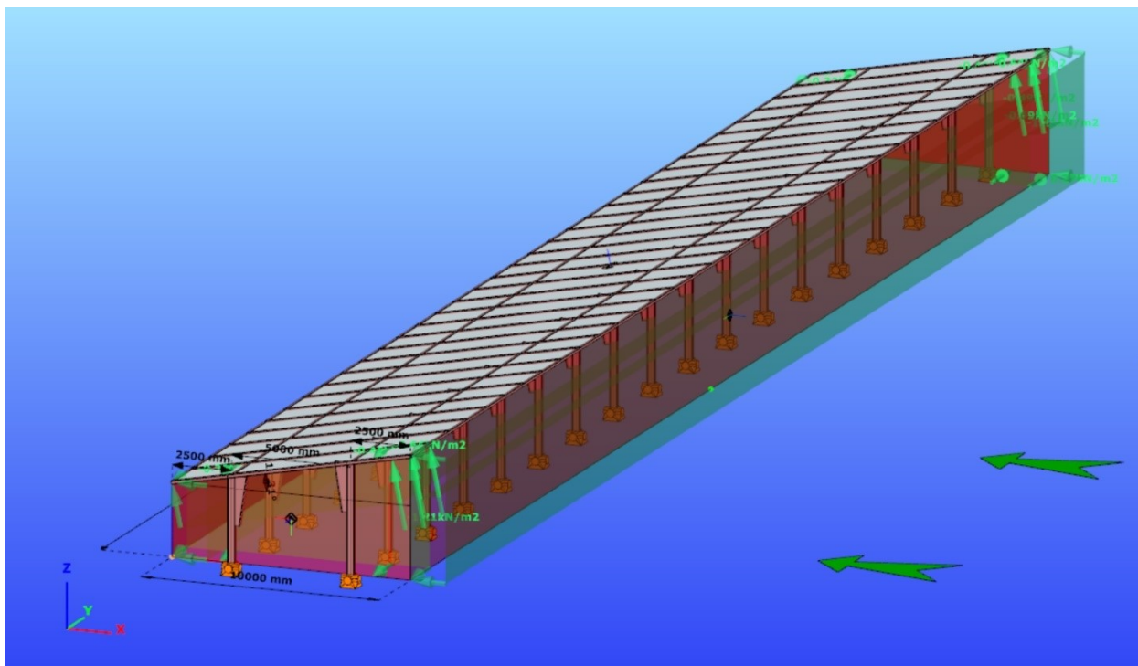
Slika 3. 5 Opterećenje vjetrom konstrukcije sa kosim krovom
