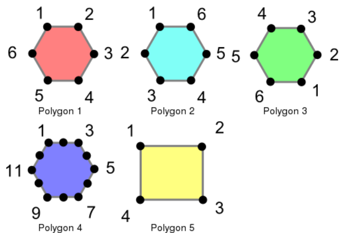
Slika 4.2 Primjeri poligona [4]
