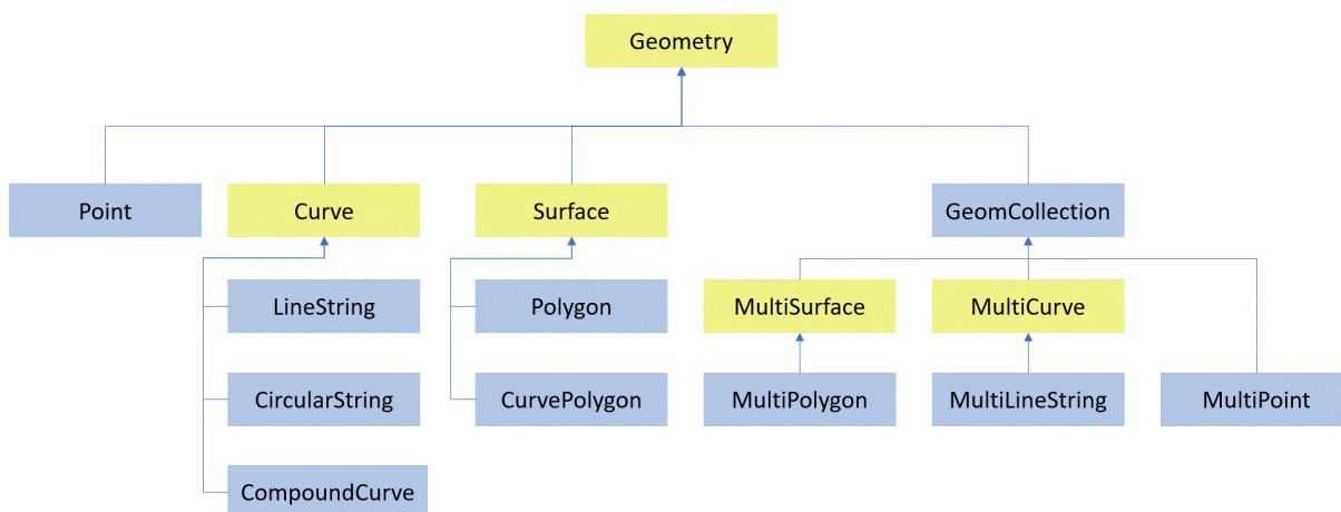
Slika 3.1 Geometrijska hijerarhija [7]
