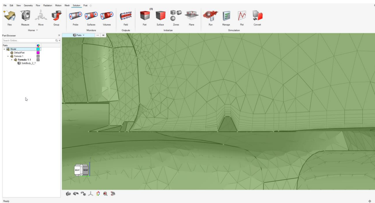
Slika 4.19. Granični dio numeričke mreže oko modela
