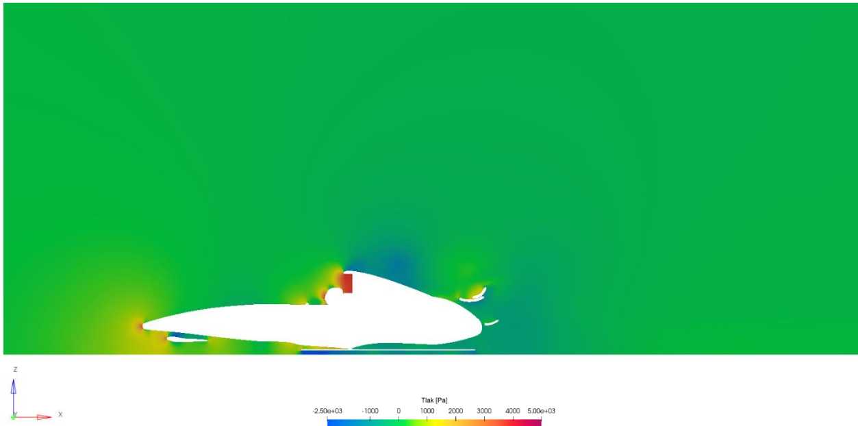
Slika 4.21. Tlak na ravnini simetrije oko automobila
