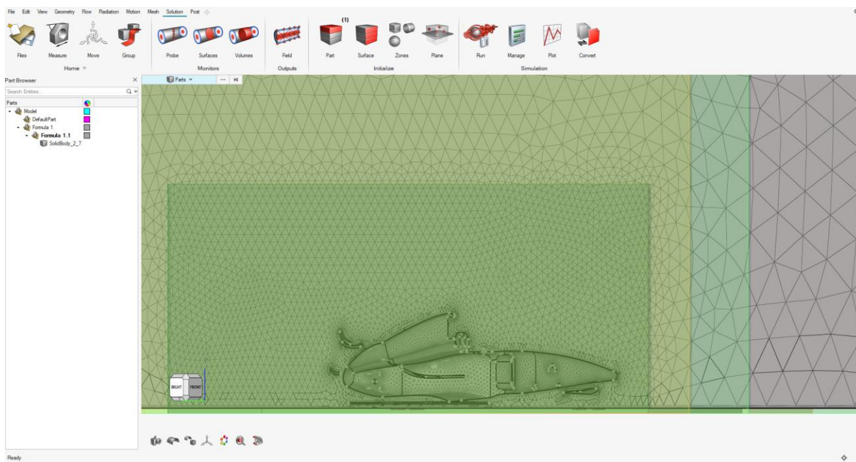
Slika 4.18. Numerička mreža domene
