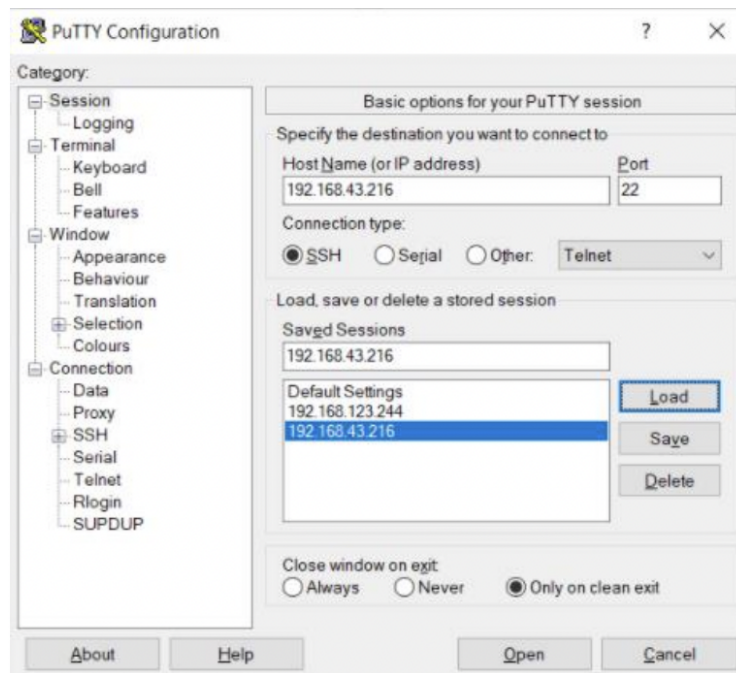
Slika 3.3.1 PuTTY konfiguracija
