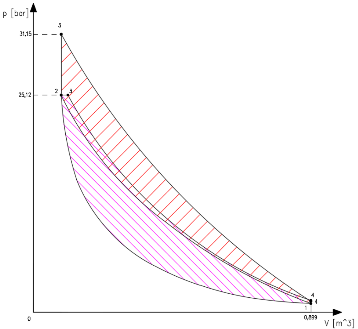
Slika 5.4. pV dijagram Ottovog i Diesellovog procesa s jednakim \varepsilon
