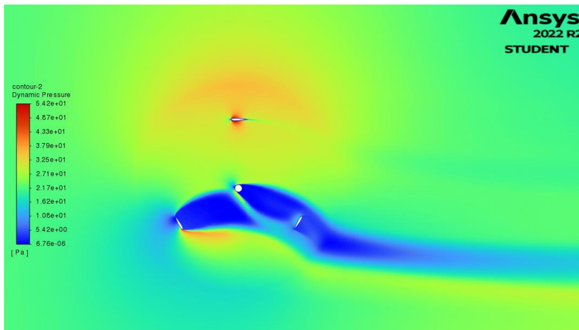
Slika 6.3 Konture dinamičkog tlaka za zakret lopatica iznosa 0°
