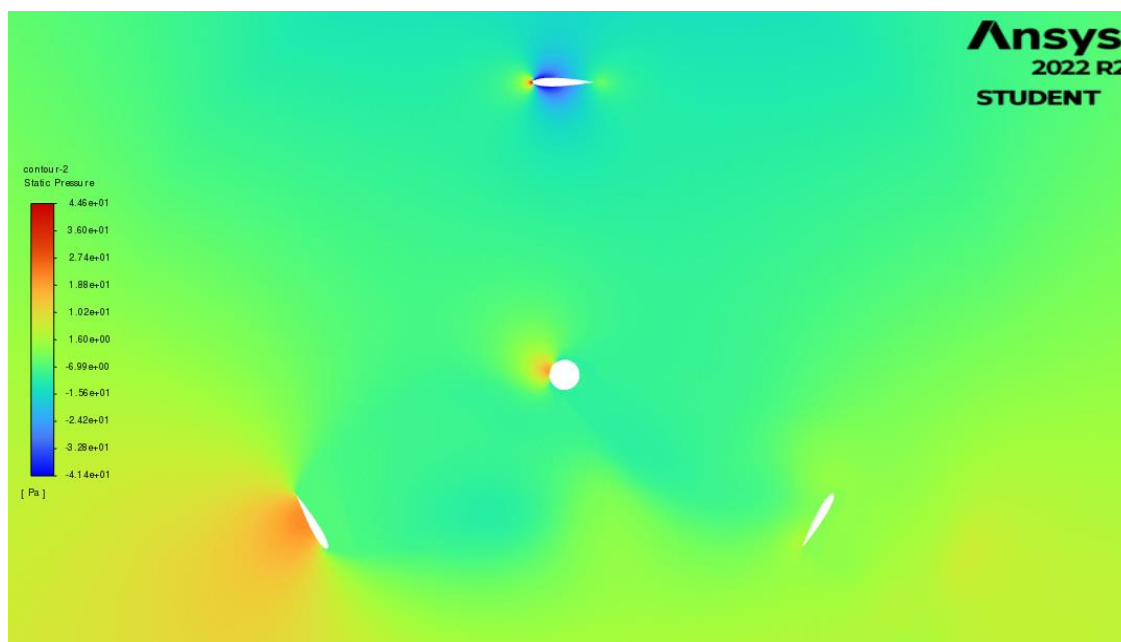
Slika 6.2 Konture statičkog tlaka za zakret lopatica iznosa 0°
