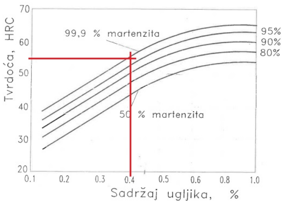
Slika 7.3. Orijentacijske vrijednosti tvrdoće čelika u ovisnosti o koncentraciji ugljika u martenzitu i udjelu martenzita u mikrostrukturi čelika [11]
