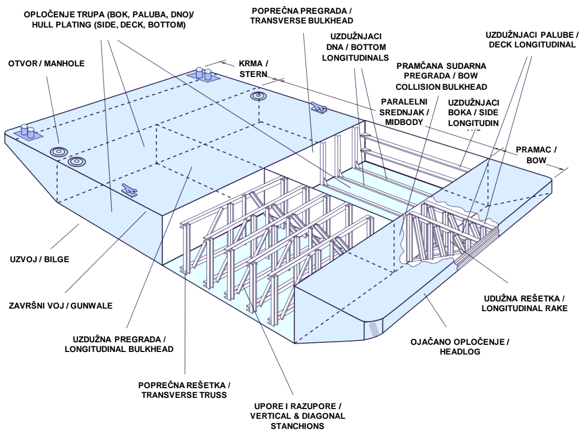
Slika 2.2. Skica primjera strukture barže za unutarnju plovidbu [3].
