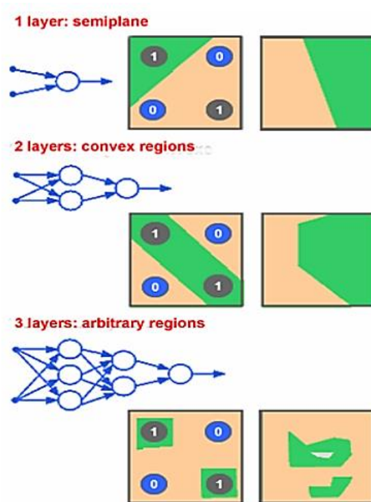
Slika 3.17. Područja odlučivanja kod višeslojnih perceptrona
