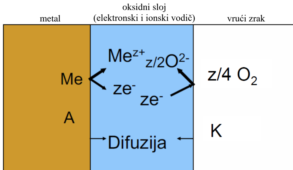
Slika 2.3. Wagnerova teorija kemijske korozije [6]
