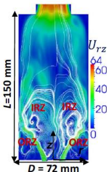
Slika 4.12. Trenutačno polje protoka turbulentnih plamenova smjese \text{NH}_3 /zrak - strujnice i dvodimenzionalna raspodjela brzine u vertikalnoj ravnini
