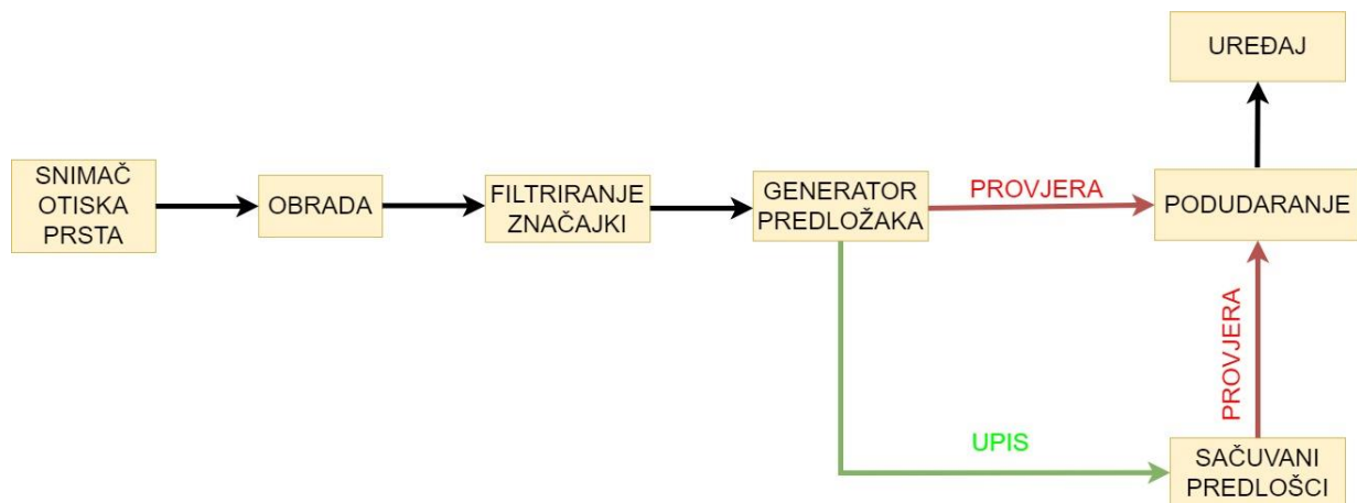
Slika 7.3. Proces autentifikacije
