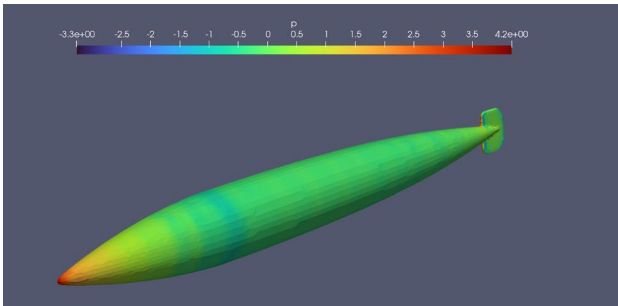
Slika 4.15. Raspodjela tlaka na trup – Siluro A.22
