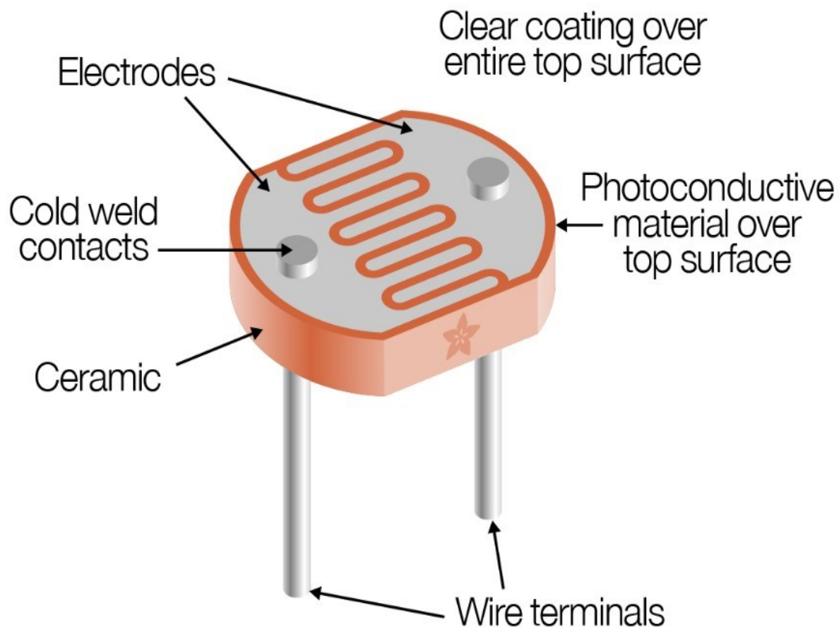
Slika 4.1: Fotootpornik [8]
