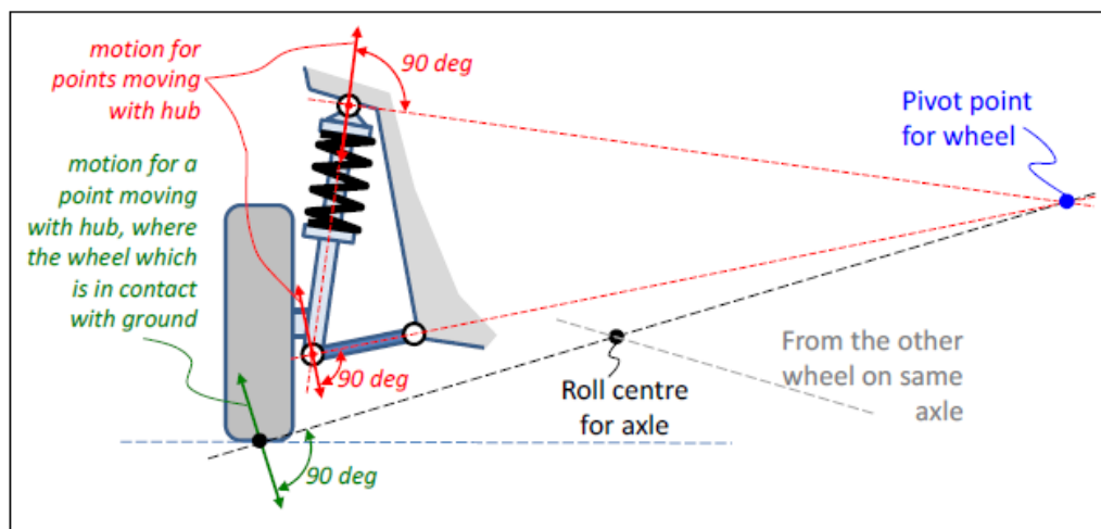
Slika 3.20 Primjer kako odrediti okretnu točku za jedan kotač i središte valjanja za osovину s dvostrukim McPhersonovim ovjesom.
