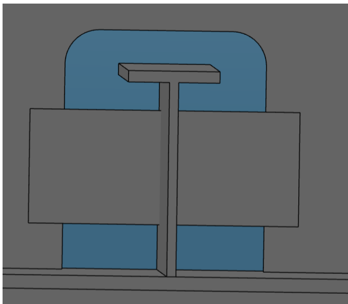
Slika 6.76. Prikaz prolaza profila „P21-TB180x8x80x10“ unutar detaljnog model broda
