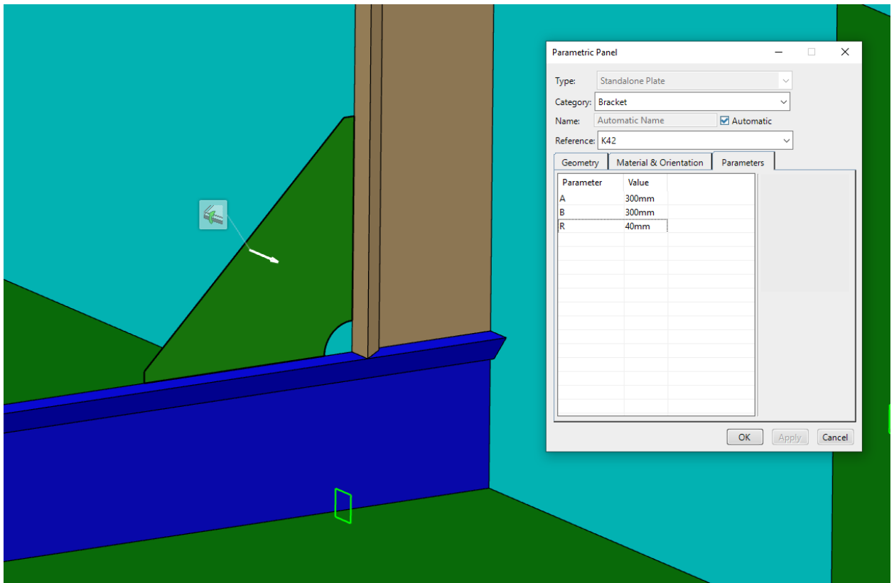
Slika 5.30. Koljeno „K42“
