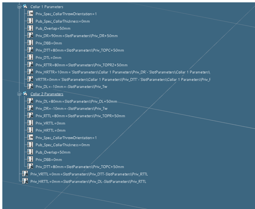
Slika 6.51. Parametri definicije konture generičkog prolaza profila „P13-FB150x10“, 3.dio
