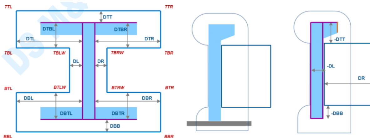
Slika 4.156. Prikaz predefiniranih parametara za definiciju konture pločice [9]
