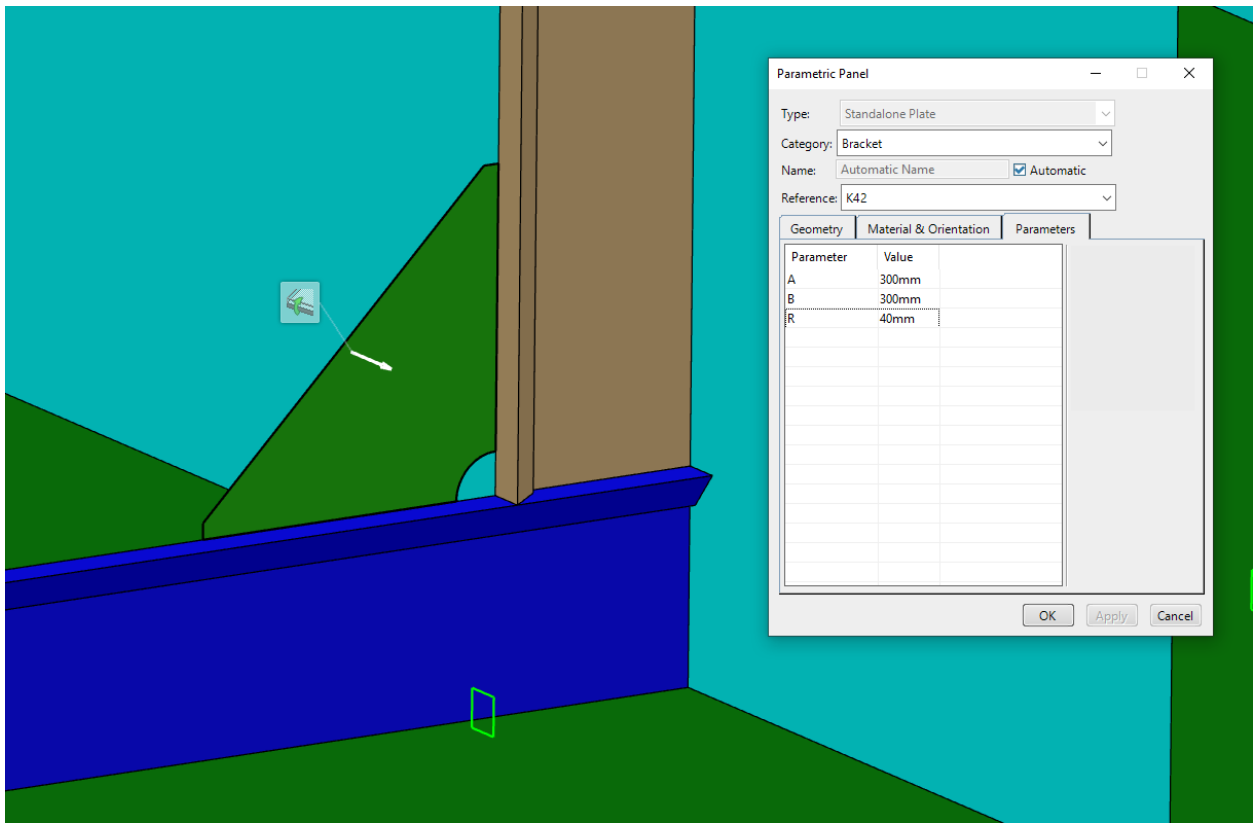
Slika 5.30. Koljeno „K42“
