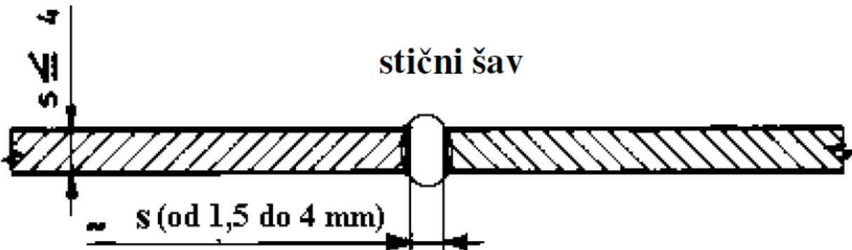
Slika 4. Stični šav
