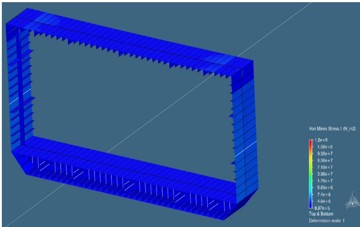
Slika 111. Presjek na 2L/3
