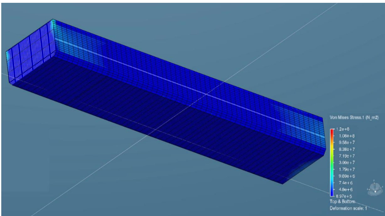
Slika 105. Von Mises naprezanja za Simulaciju 1 – Dno
