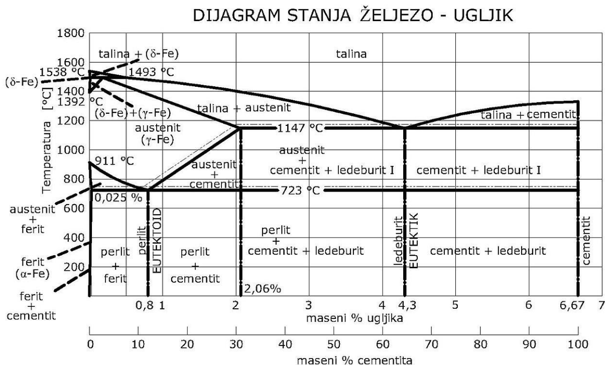
Slika 2.12. - Fe-Fe 3 C dijagram [11]
