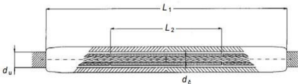
Slika 4.3.1. Dimenzije nastavne kompresijske spojnice [6]
