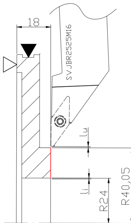
Slika 5.38. Operacija 40 – zahvat 4
