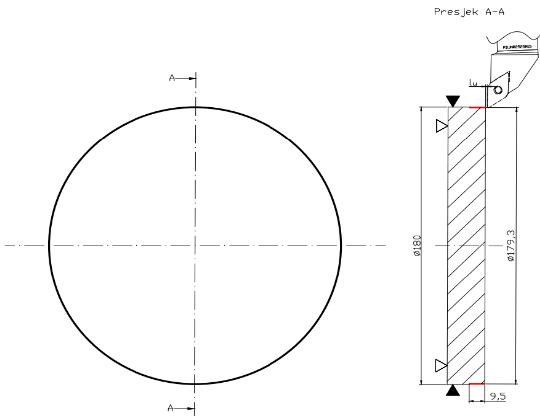
Slika 5.10. Operacija 20 – zahvat 3
