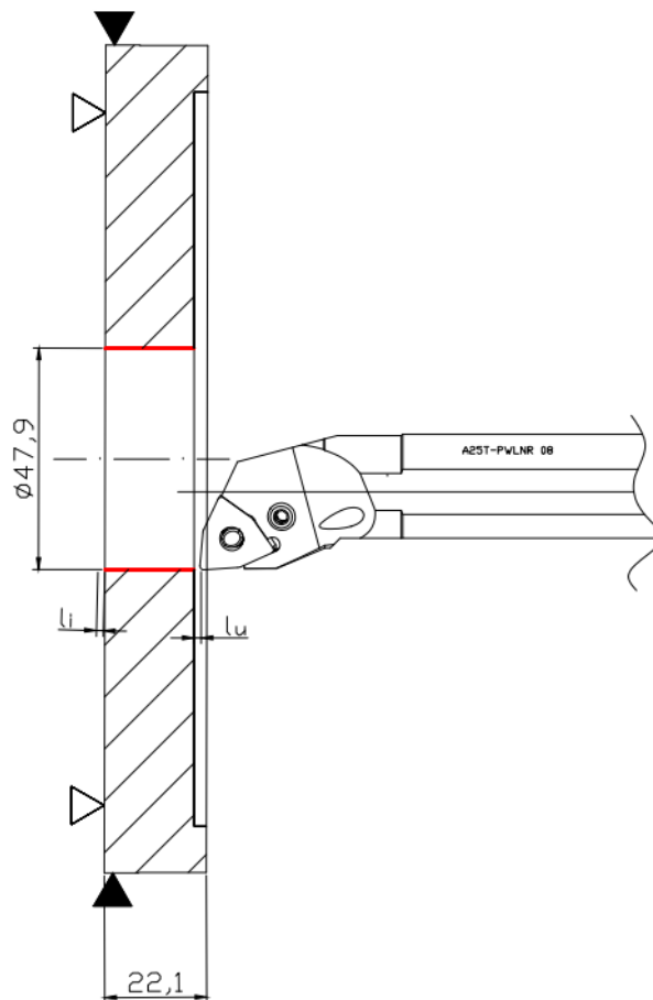
Slika 5.21. Operacija 30 – zahvat 5
